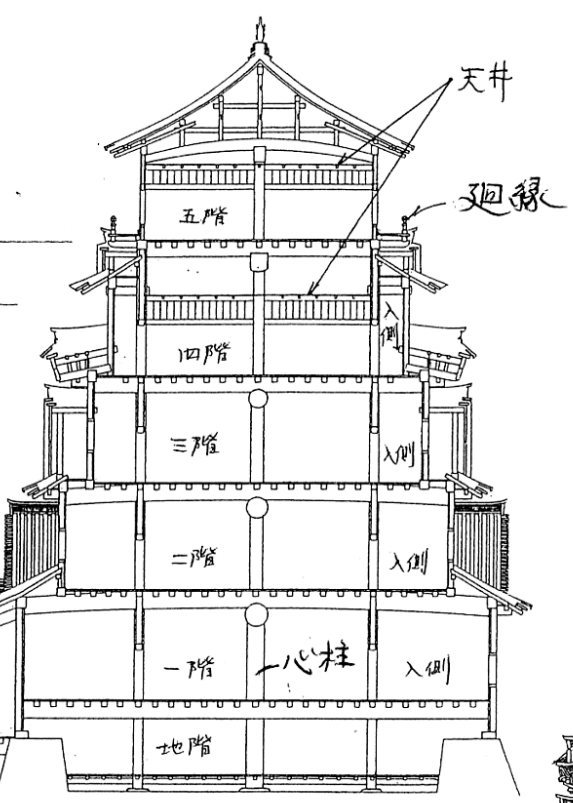
南北断面図
